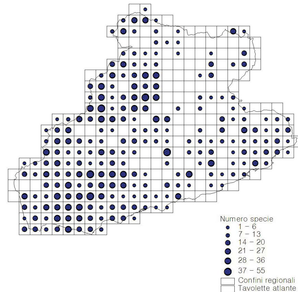
Figura 2. Copertura ottenuta con i dati raccolti nel 2005 e 2006 (235 tavolette che rappresentano il 70,7% della copertura provinciale).
