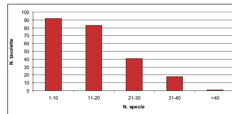
Figura 3. Grafico del numero tavolette/numero specie
