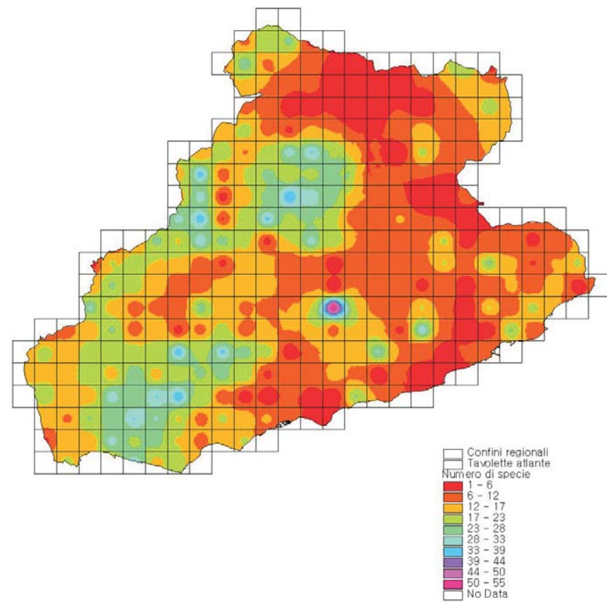
Figura 3. Carta interpolata della ricchezza di specie.
