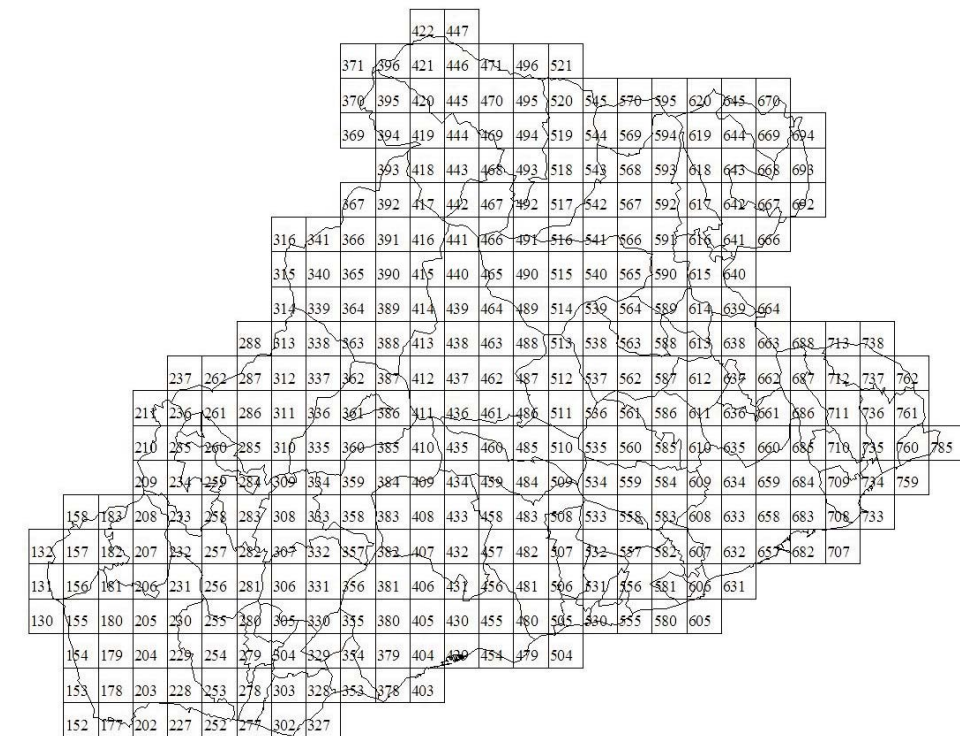
Figura 1 . Griglia di rilevamento di 2 km di lato.
